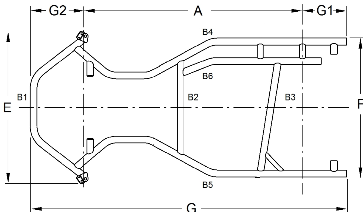
VUE DE DESSUS / VIEW FROM ABOVE
