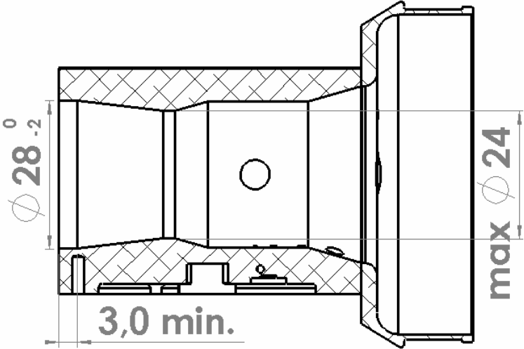
DESCRIPTION DU CARBURATEUR ET ESQUISSE DES PIÈCES
