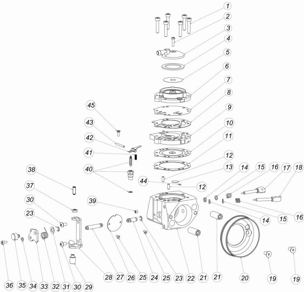
DESCRIPTION DU CARBURATEUR ET ESQUISSE DES PIÈCES
