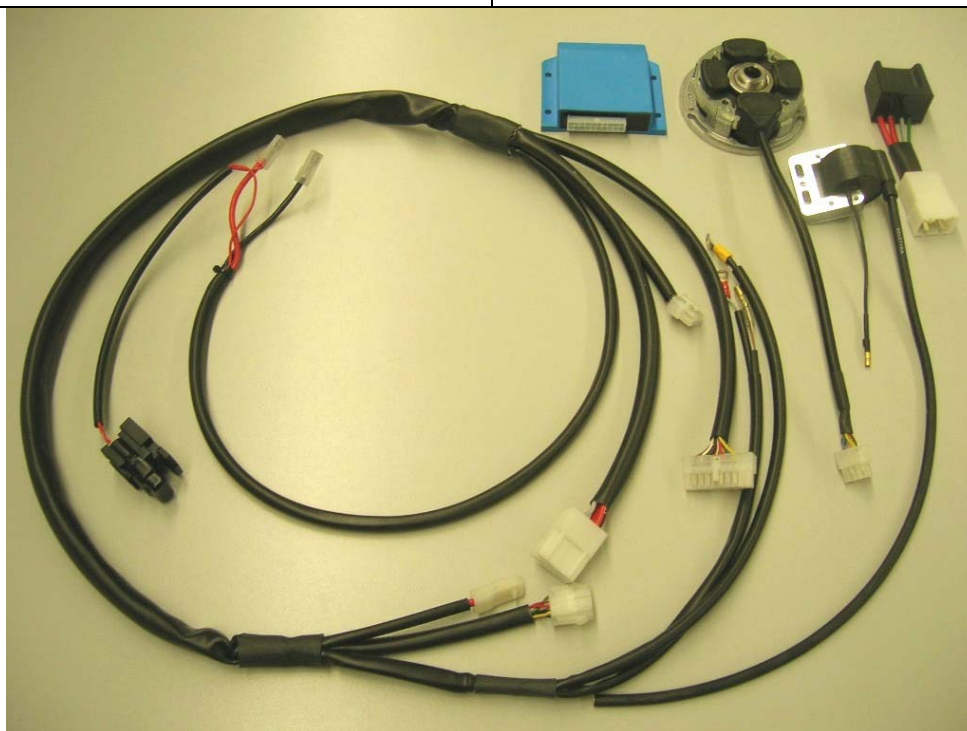
PHOTO de l'ensemble rotor, stator, bobine, boîtier électronique et cablage complet
